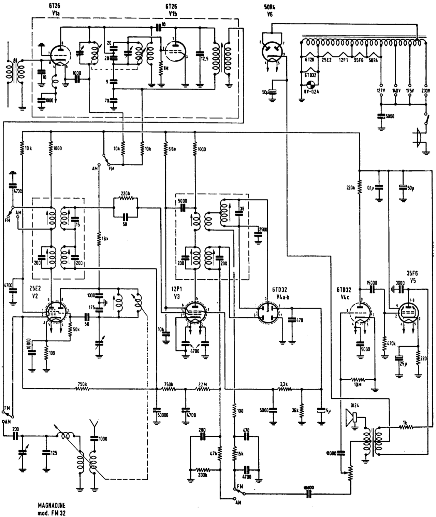
SCHEMA ELETTRICO DEL RADIORICEVITORE AM-FM, MAGNADINE, MOD. FM32
